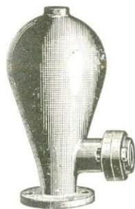
Fig. 8 Récipient à sortie latérale
