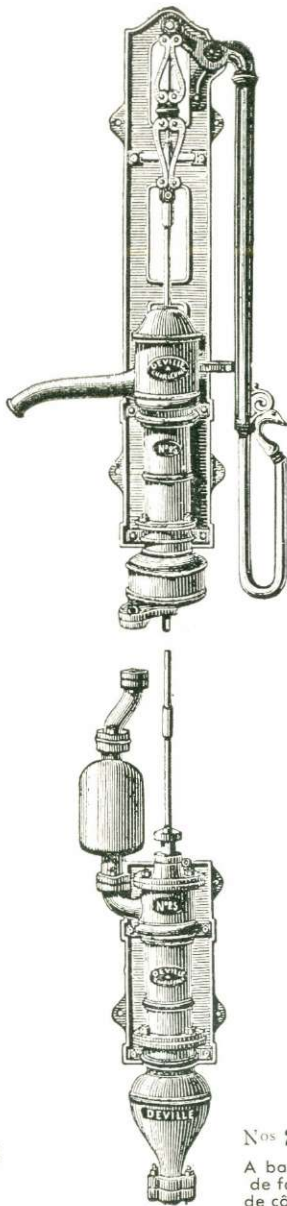
N os 93, 94 Bornes sur pieds à volant
