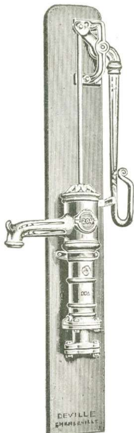
à balancier de côté avec ou sans aiguille (Modèle sans aiguille)
