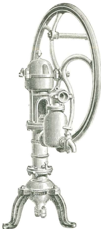
Aspirante et foulante borne sur pieds N o 20
