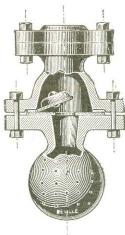
Crépine avec soupape de retenue
