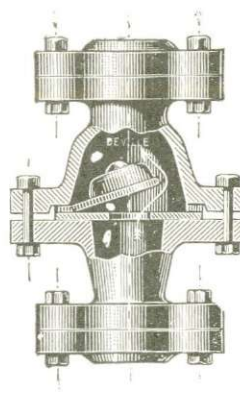
Soupape de retenue
